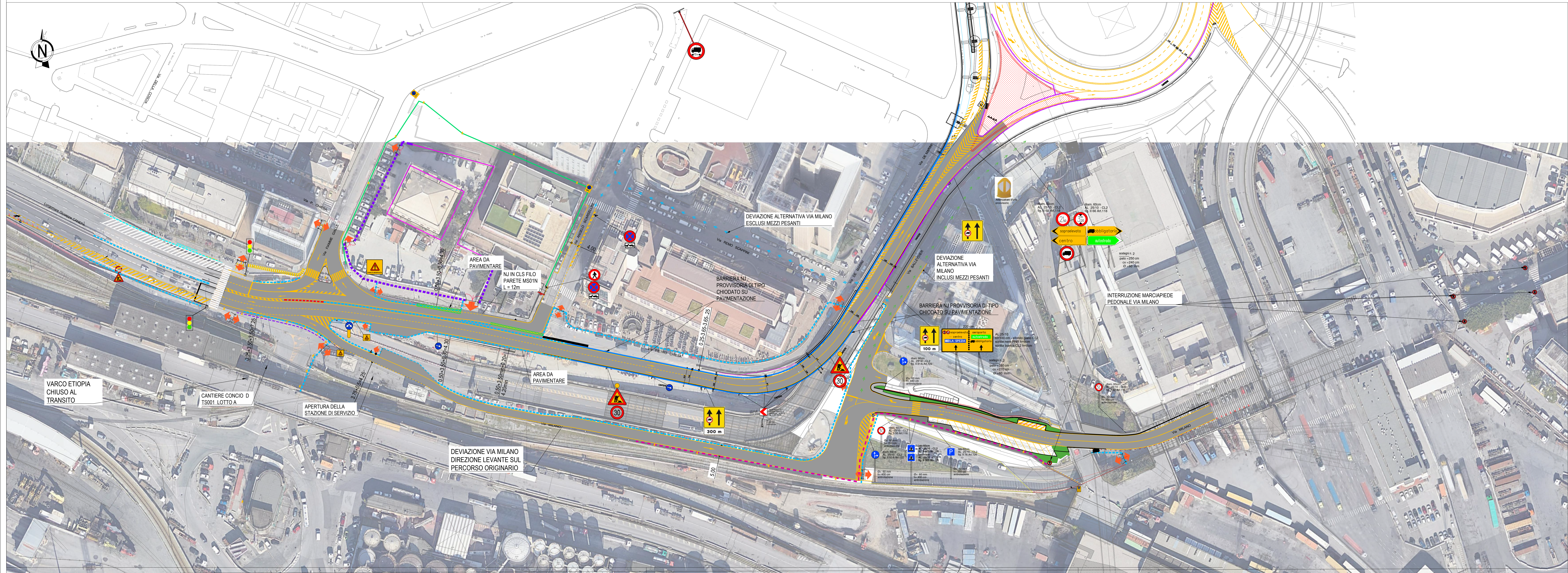
PLANIMETRIA CANTIERIZZAZIONE VIABILITA' LUNGOMARE CANEPA - VIA MILANO DIREZIONE LEVANTE scala 1:500
