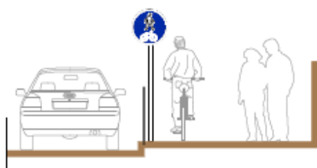
VIA GIOTTO doppio senso unico dir. ponente su marciapiede esistente percorso ciclopeditonale TIPOLOGIA GIO 2
