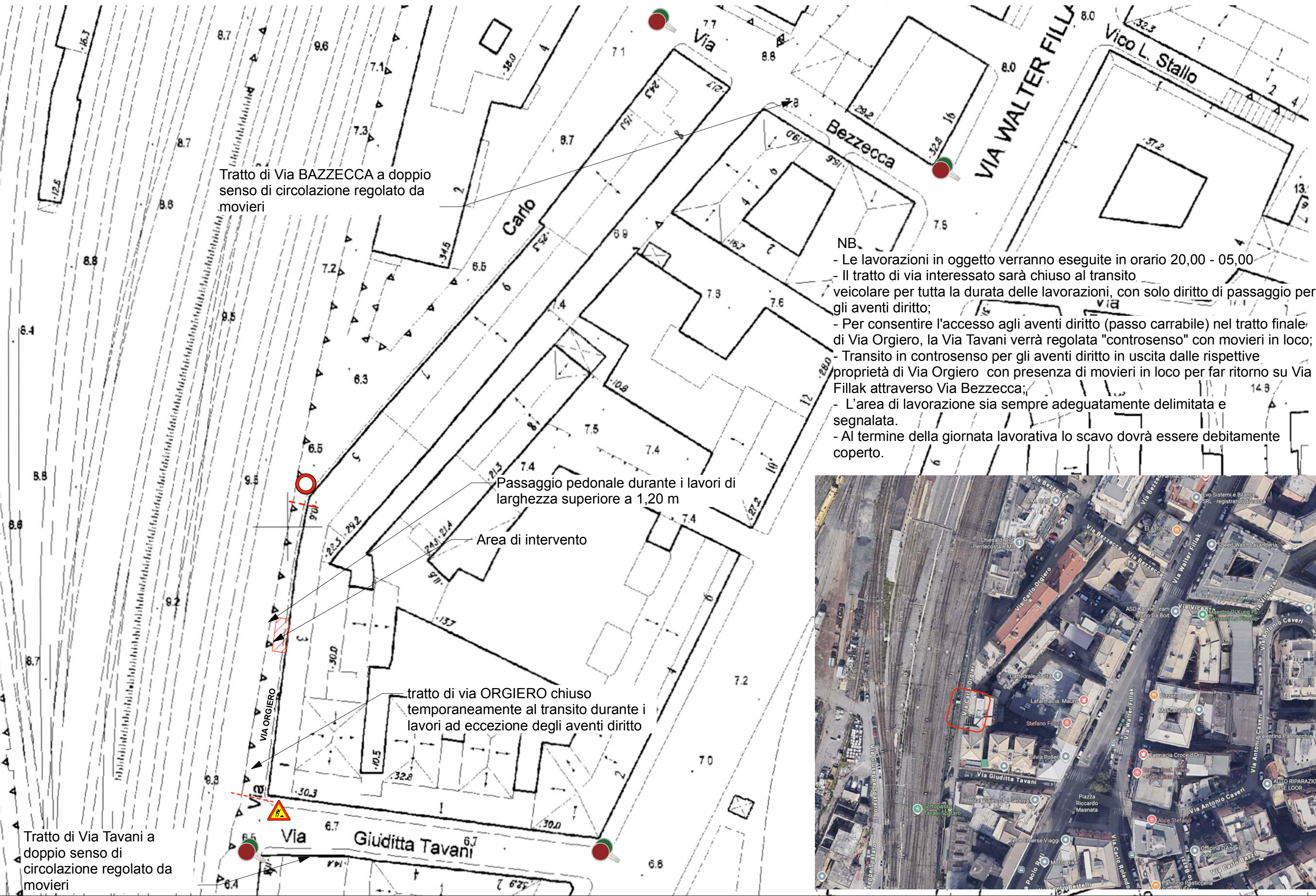
PLANIMETRIA AREE DI CANTIERE VIA ORGIERO
