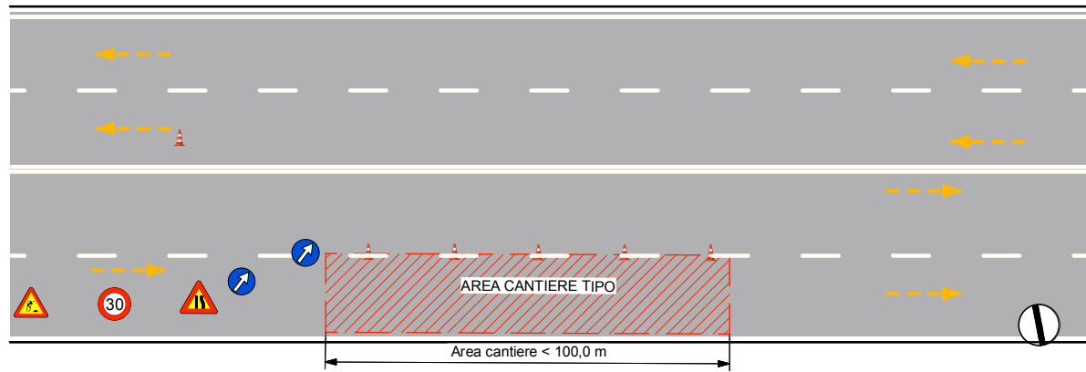
Schema tipologico con segnaletica e transito su via Buozzi
