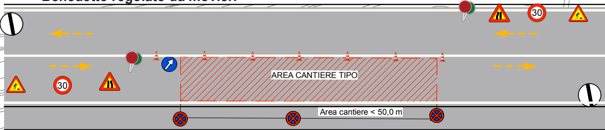
Schema tipologico con segnaletica e transito a senso unico alternato su via S. Benedetto regolato da movieri
