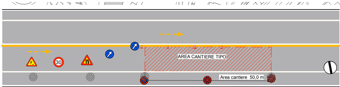
Schema tipologico segnaletica e transito a senso unico su via di Francia
