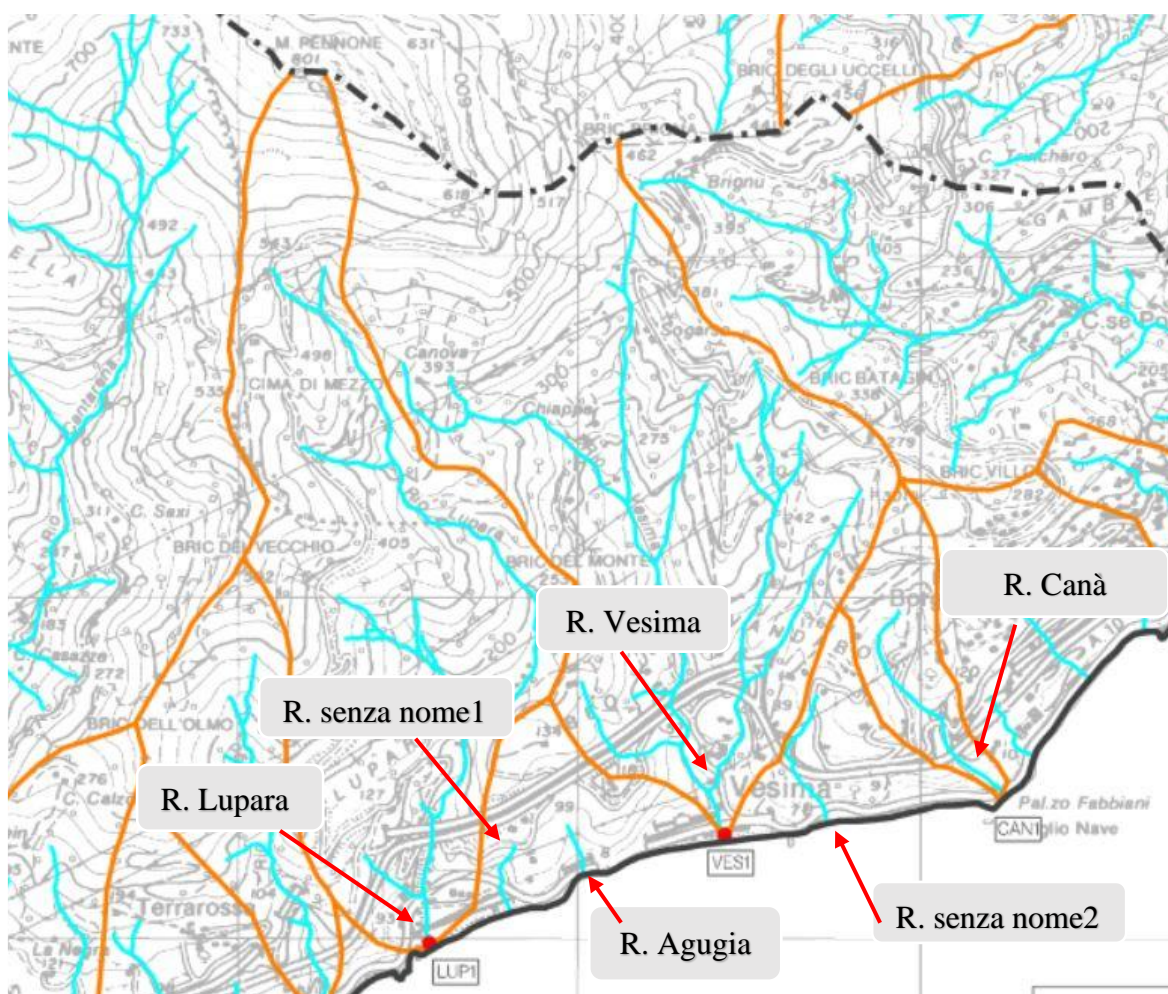
Figura 4: Estratto della Carta del reticolo idrografico del P.d.b.
