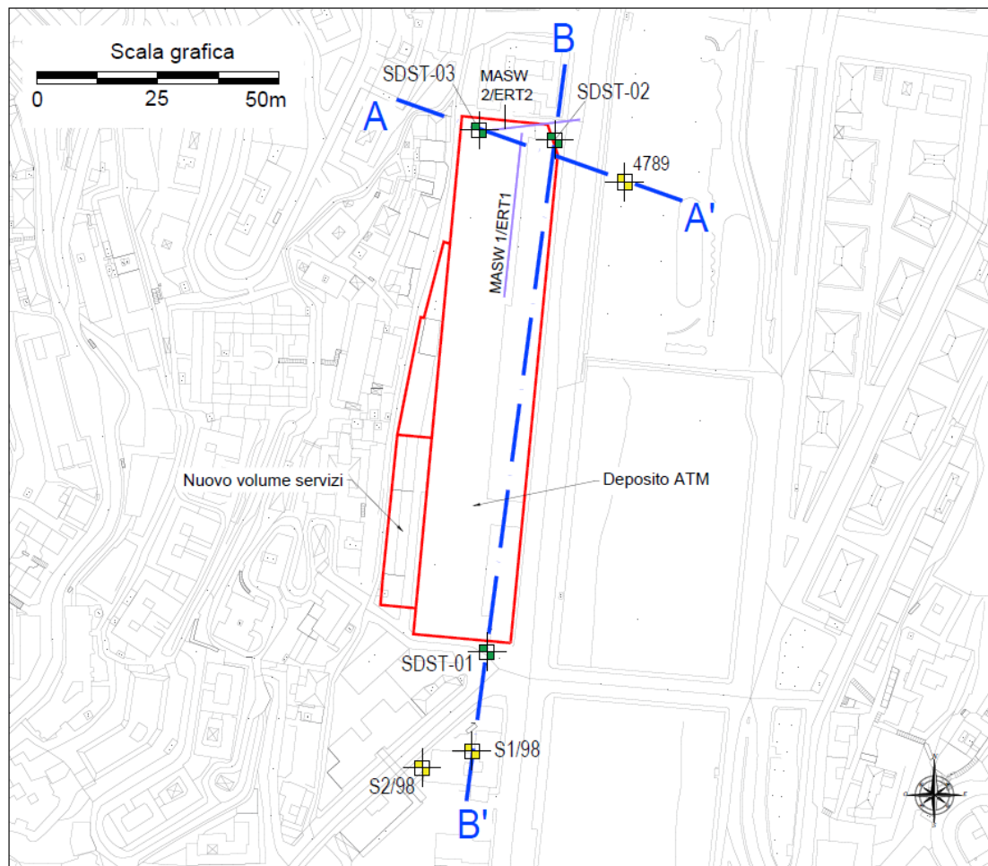
Figura 18 Pianta su base topografica con indicazione delle prove in sito e dell'ingombro dei nuovi edificati. In blu la traccia dei profili geotecnici eseguiti.
