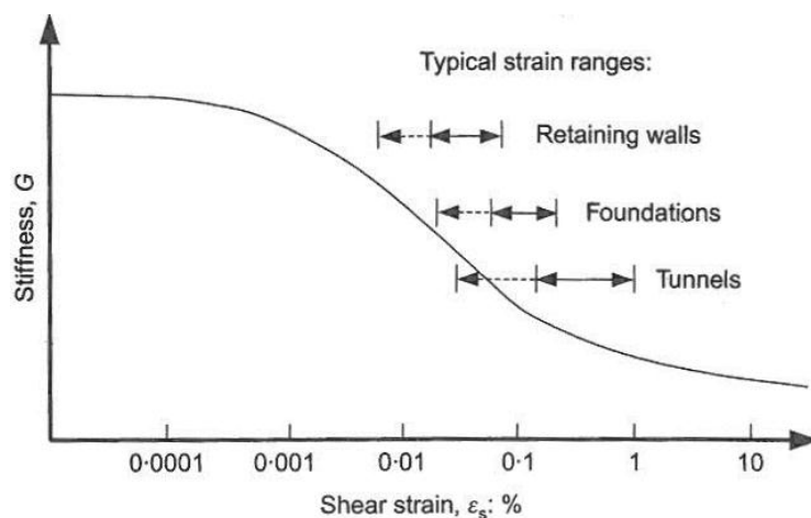
Figura 8: Variazione tipica del modulo di rigidità in funzione della deformazione unitaria, Mair (1993).
