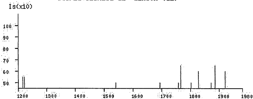
Storia sismica di GENOVA (GE)
