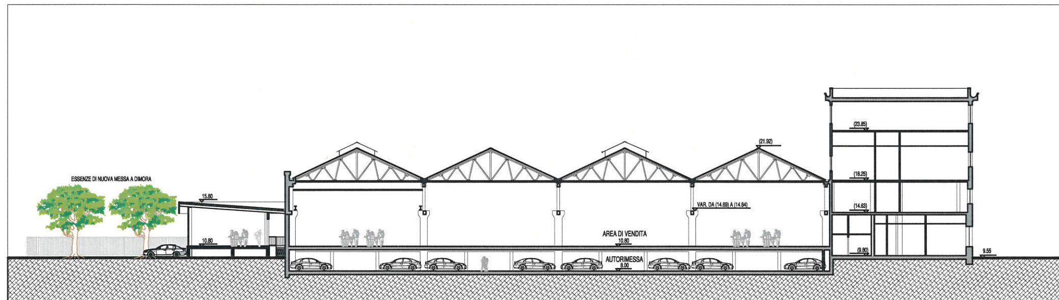
SEZIONE TIPOLOGICA TRASVERSALE Stato Attuale COINCIDENTE con Stato Finale - NON OGGETTO DI INTERVENTI
