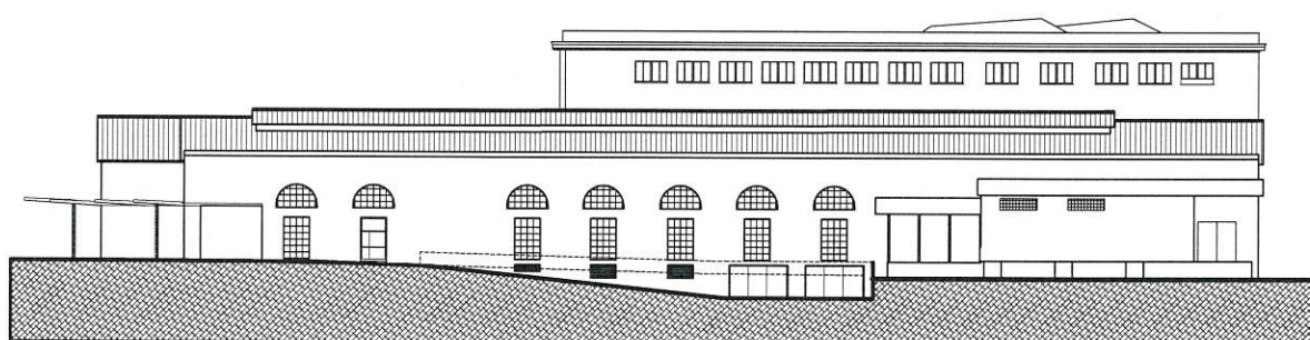
PROSPETTO EST Stato Attuale COINCIDENTE con Stato Finale - NON OGGETTO DI INTERVENTI
