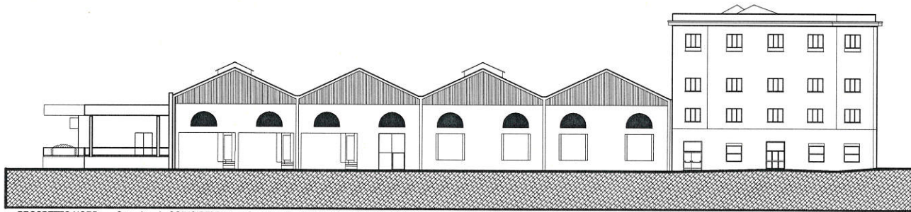
PROSPETTO NORD Stato Attuale COINCIDENTE con Stato Finale - NON OGGETTO DI INTERVENTI
