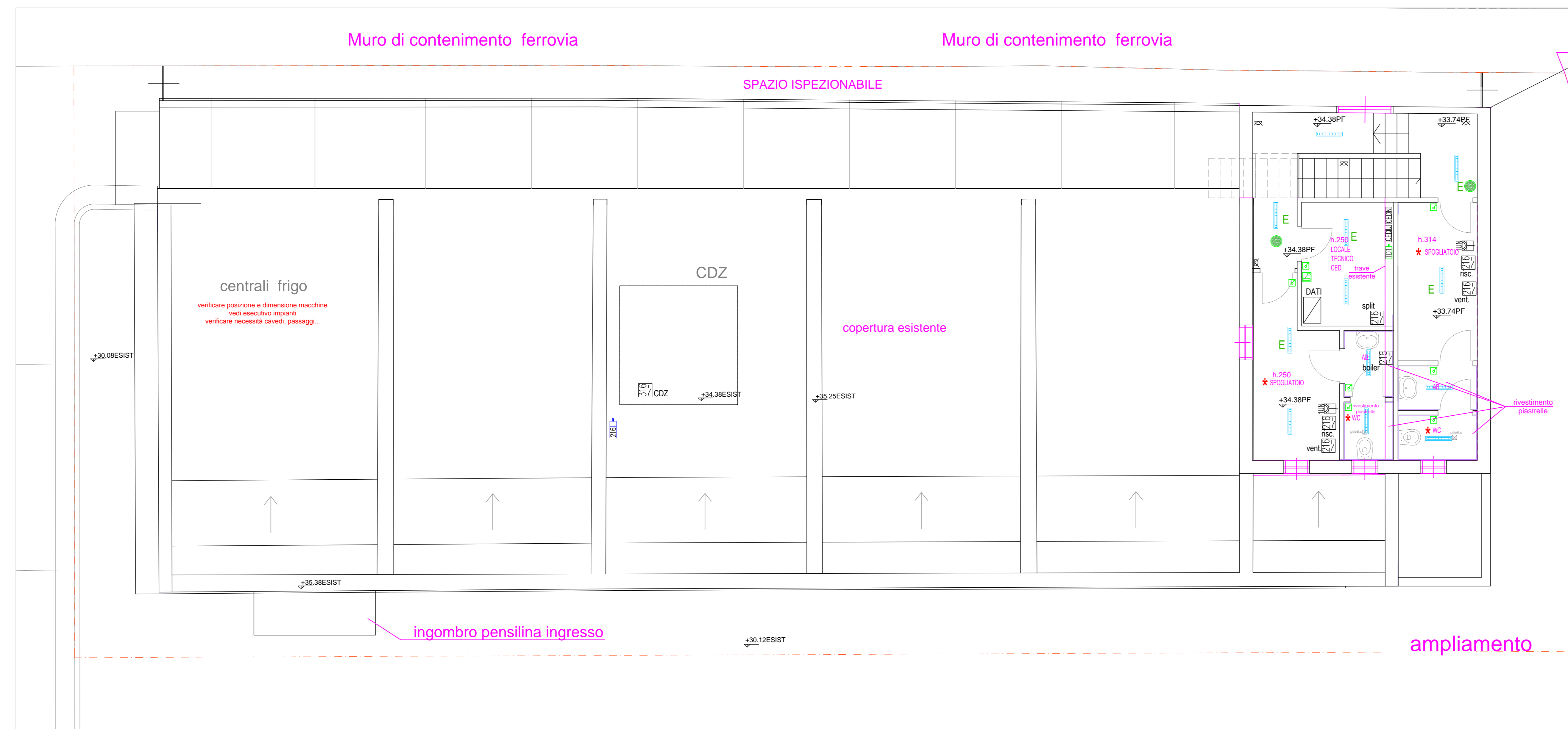
PIANTA Quota +35.50
